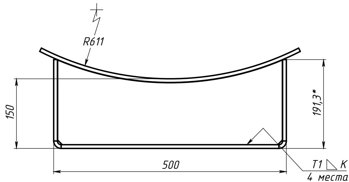
Поз.3 (Ложмент)
