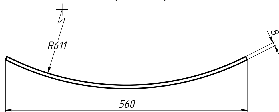
Поз.3 (Ложмент)
